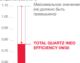
Тест на бензиновом двигателе 1,8 л* Степень износа (нм/ч)
