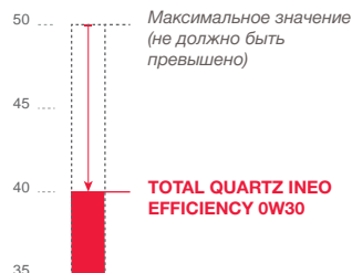
Тест на 3-литровом бензиновом двигателе* повышение вязкости при 100°C
