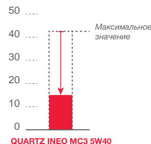
ТЕСТ НА ДИЗЕЛЬНОМ ДВИГАТЕЛЕ Износ кулачков - в среднем (µm)
