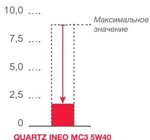
ТЕСТ НА БЕНЗИНОВОМ ДВИГАТЕЛЕ Износ кулачков - в среднем (µm)
